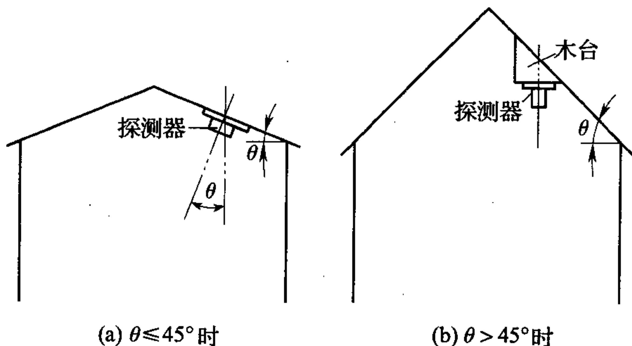
图 6 探测器的安装角度
