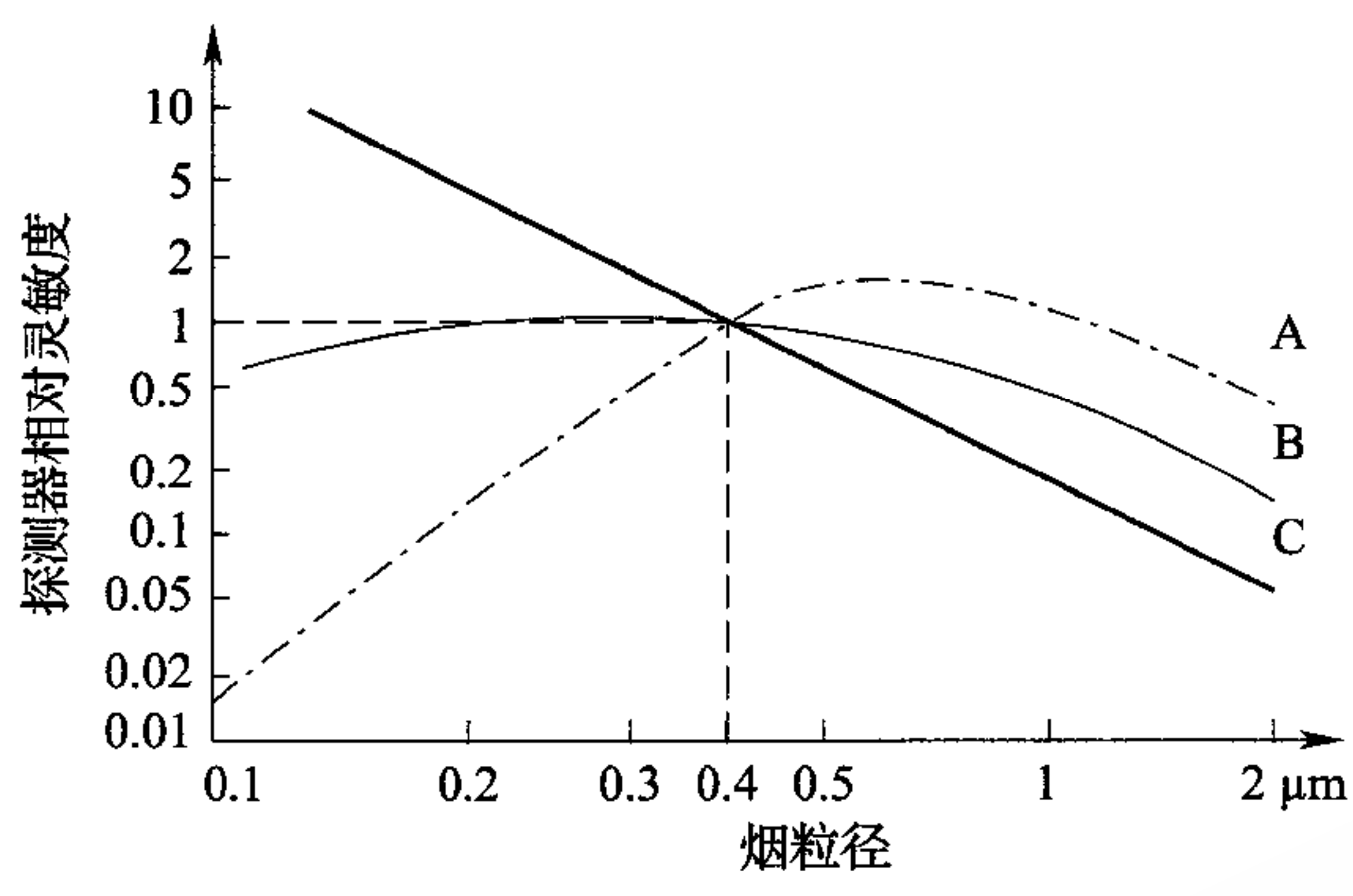
图 2 感烟火灾探测器对不同烟粒径的响应 A—散射型光电感烟火灾探测器；B—减光型光电感烟火灾探测器； C—离子感烟火灾探测器
