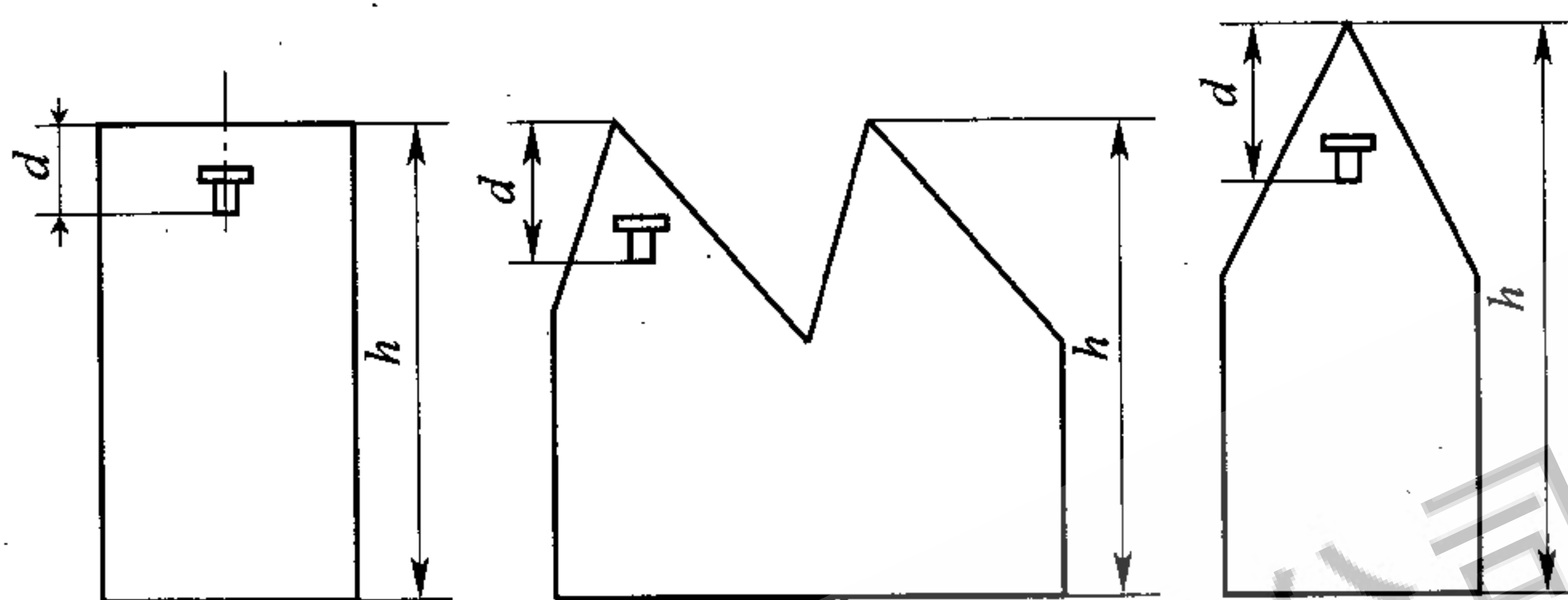
图 5 感烟探测器在不同形状顶棚或屋顶下其下表面至顶棚或屋顶的距离 d
