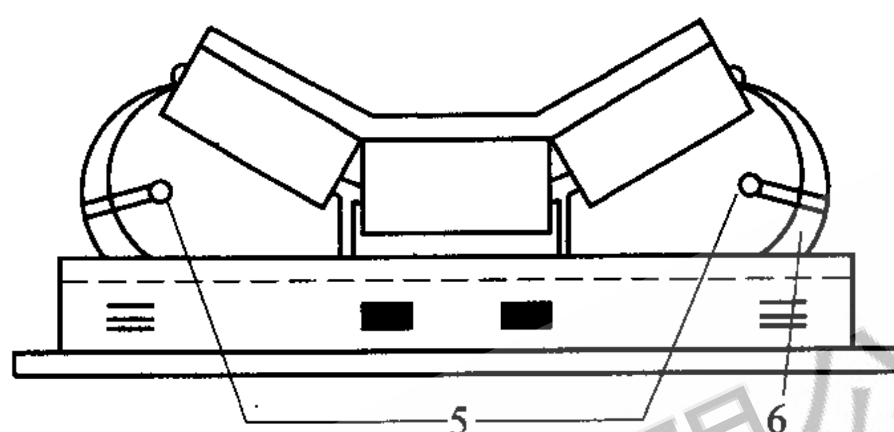
(b) 正视图
